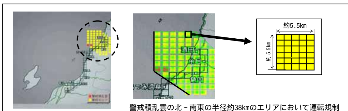
【図2】気象情報の活用による運転規制範囲のイメージ
